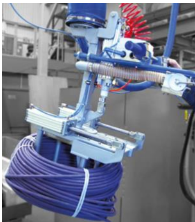
Kabelrollen Kombiniert mit pneumatischen Greifern
